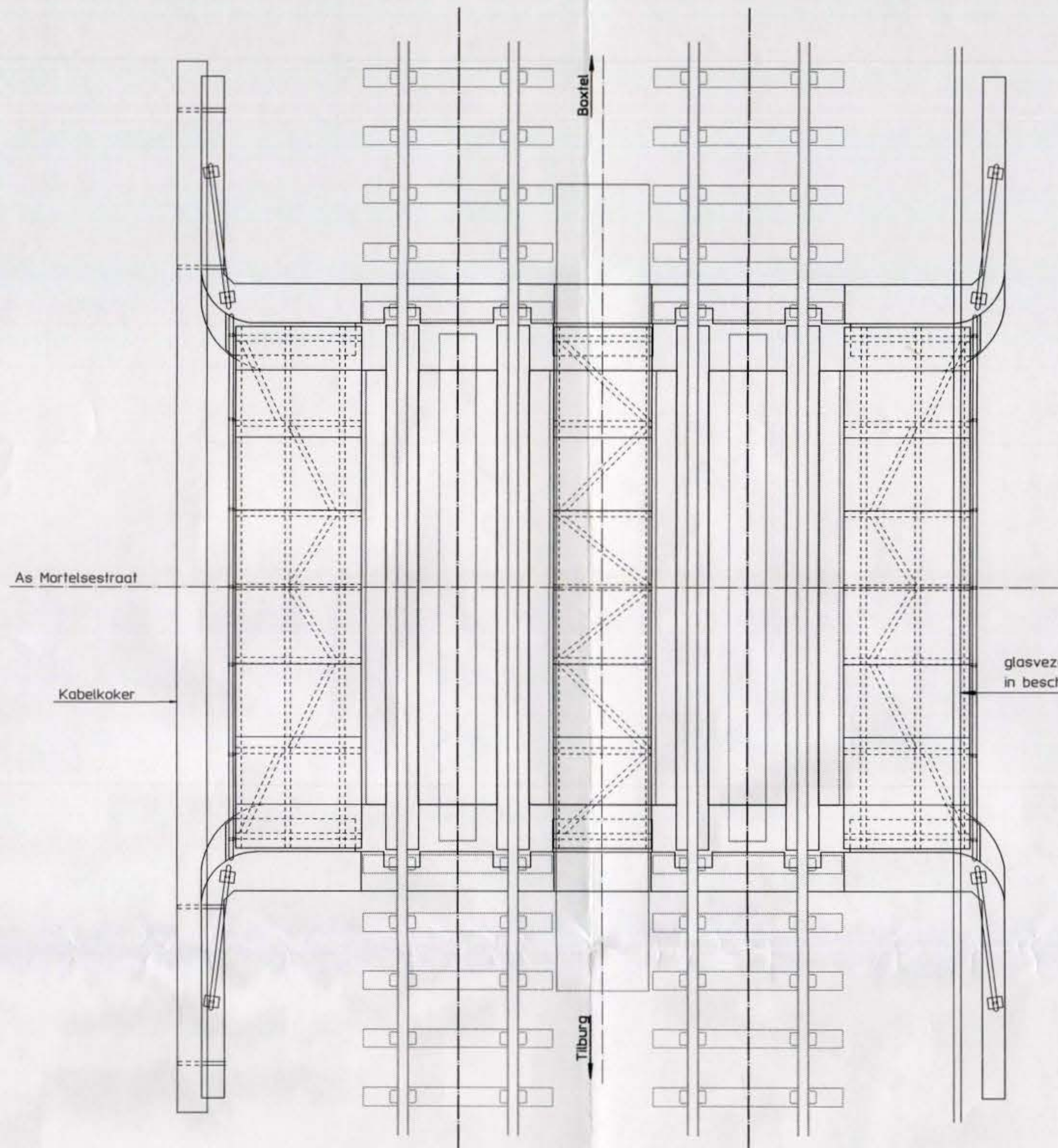
Bovenaanzicht, bestaande situatie 150
