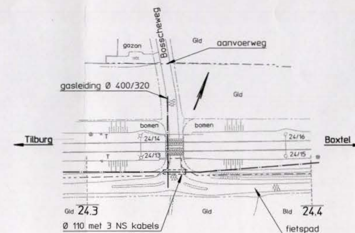
Situatie 1:1000
