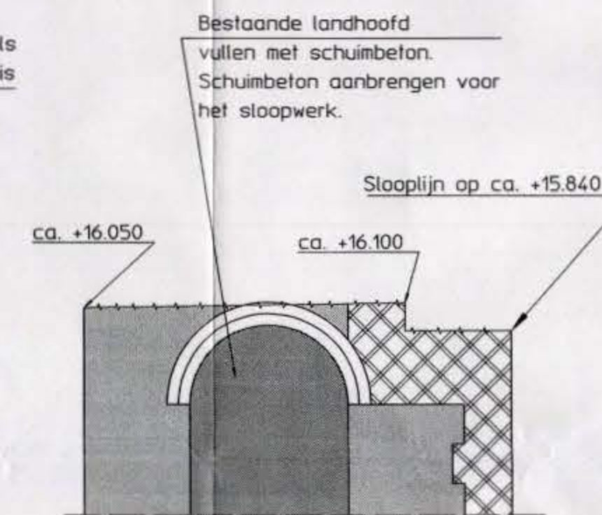
Doorsnede over landhoofd sloopvlak 150
