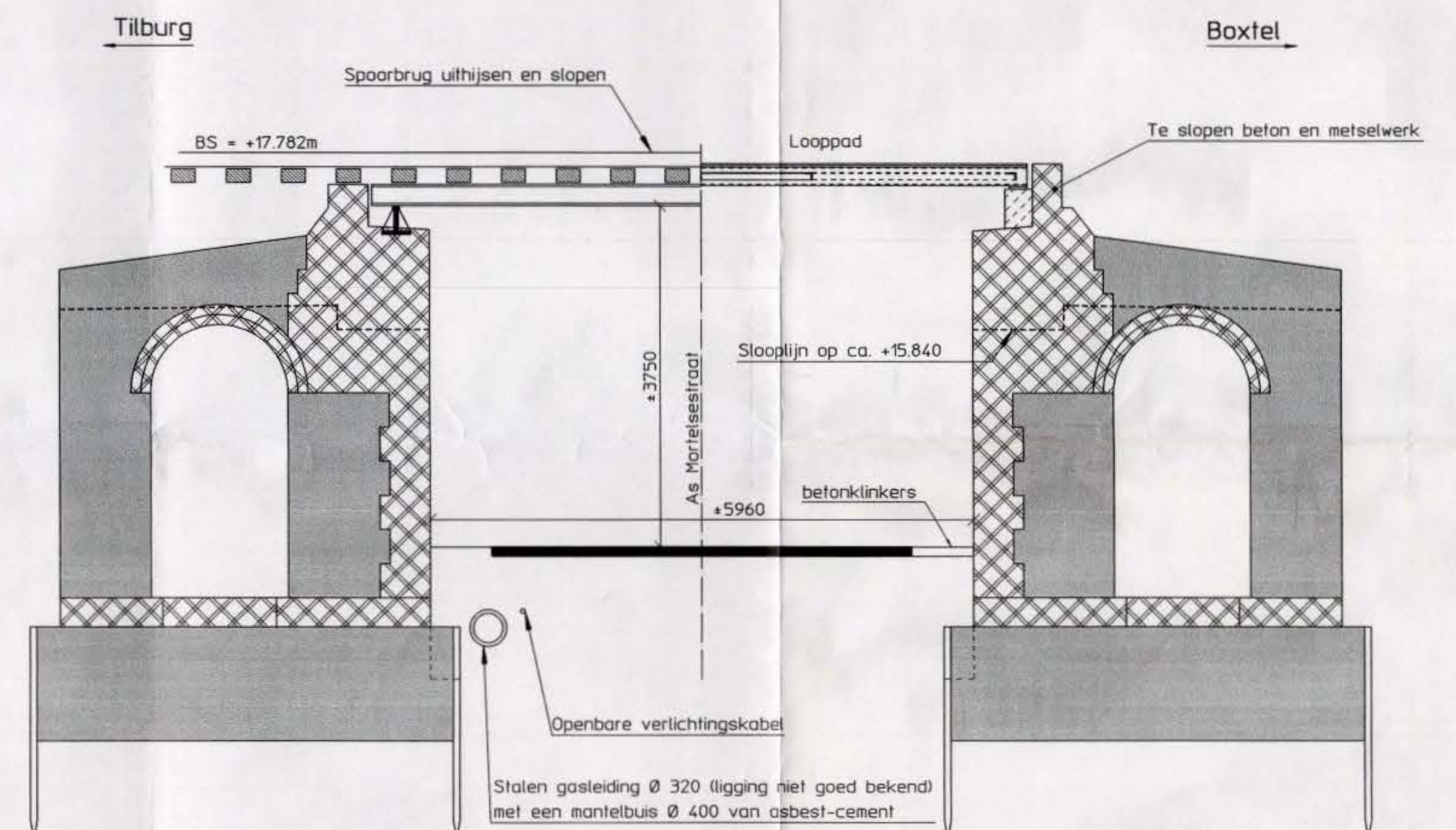
Doorsnede over as spoorbaan, bestaande situatie 150
