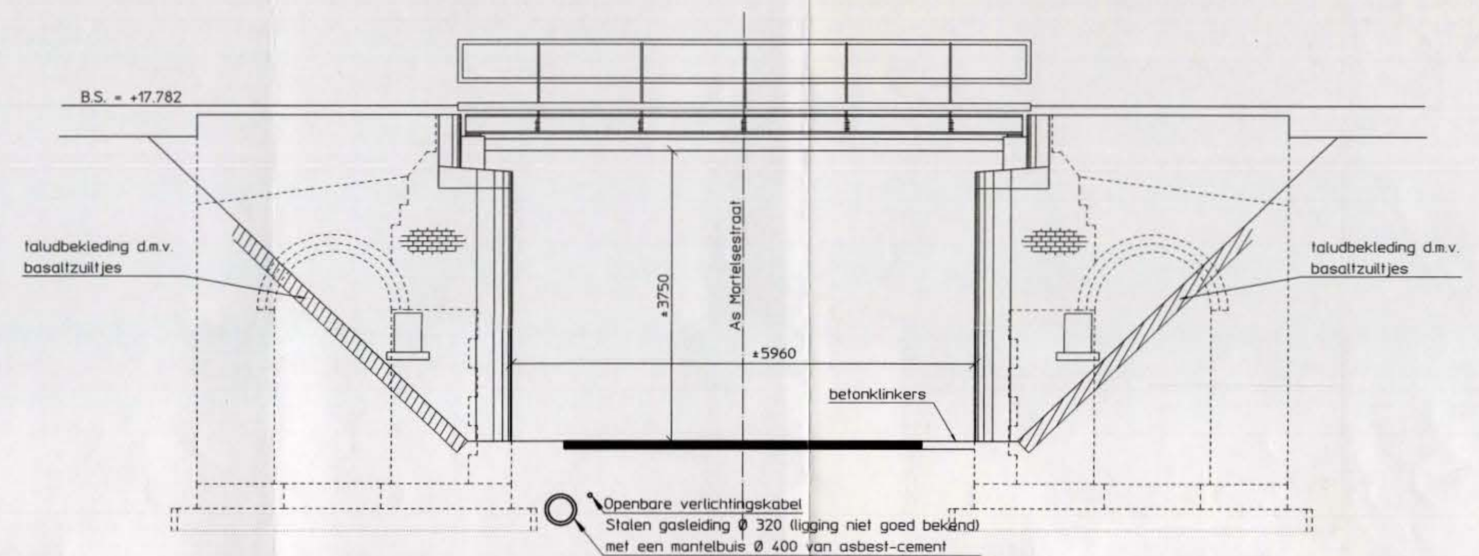
Vooraanzicht, bestaande situatie 150
